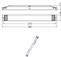
Specificationer Osram OTI DALI 90/220-240/700D LT2L VS20
